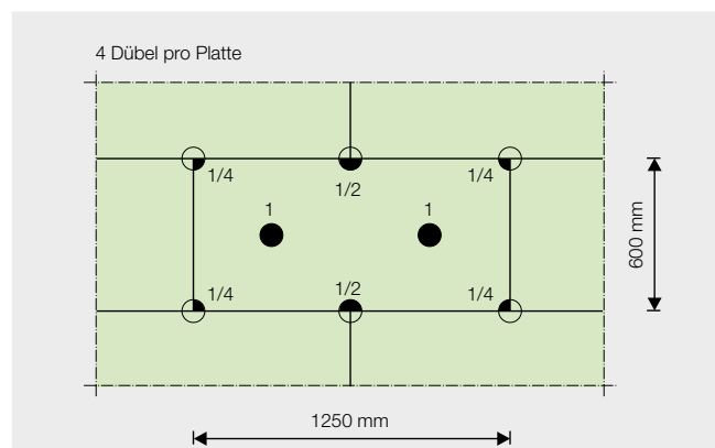
Abb. 15: Dübelanzahl (4 Dübel pro Platte) und Dübelanordnung bei nachträglicher Befestigung von Styrodur-Platten im Sockelbereich (Maße in mm)
