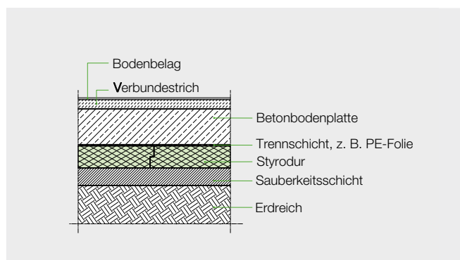
Abb. 3: Unterer Raumabschluss mit untenliegender Wärmedämmschicht, an das Erdreich grenzend
