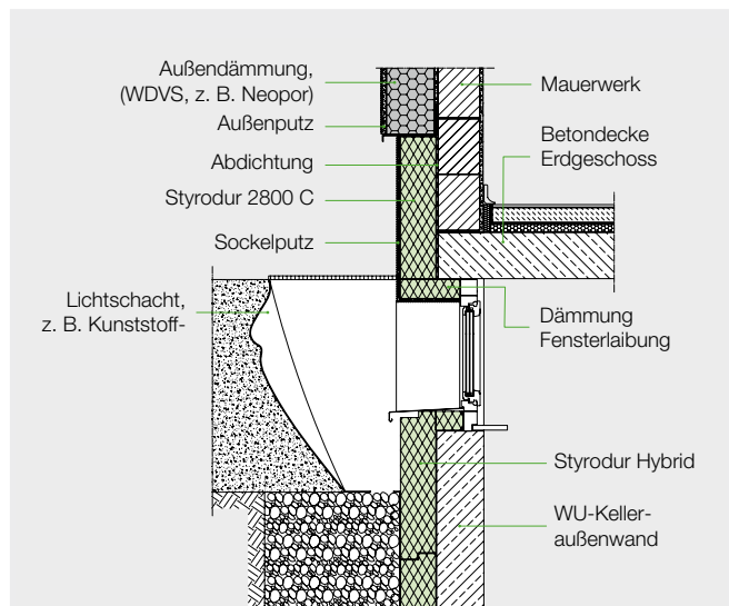
Abb. 12: Wärmebrückenfreier Anschluss eines Kunststofflichtschachtes
