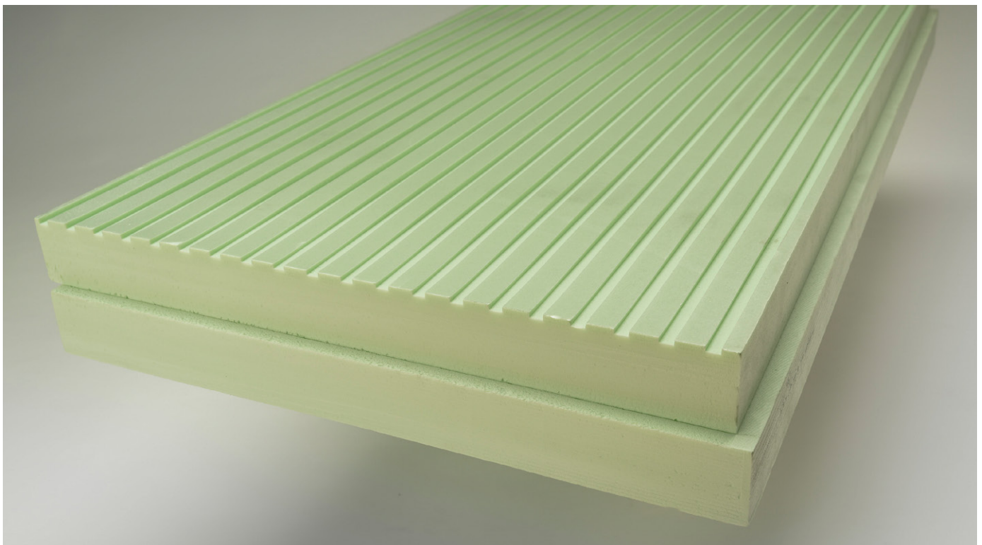
Abb. 1: Styrodur Hybrid-Platte mit Längsrillen auf einer Oberflächenseite und umlaufendem Stufenfalz
