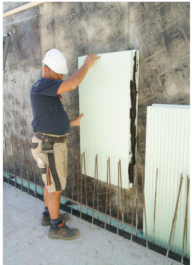
Abb. 7: Ansetzen der Styrodur Hybrid-Platten
