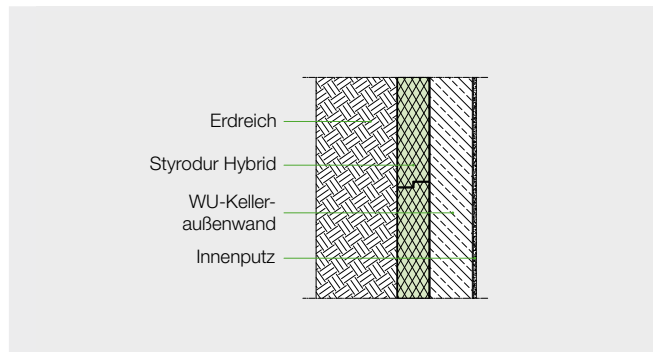
Abb. 2: Kellerwand mit außenliegender Wärmedämmschicht, an das Erdreich grenzend
