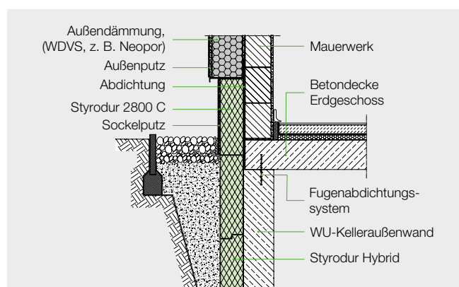
Abb. 14: Sockelbereich, Perimeterdämmung mit außenliegendem Wärmedämmverbundsystem.
